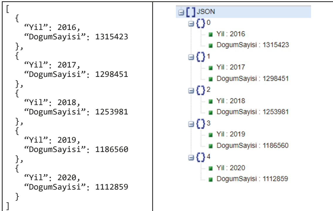
Görsel 3.2: Json dosya içeriği ve veri yapısının görünümü
